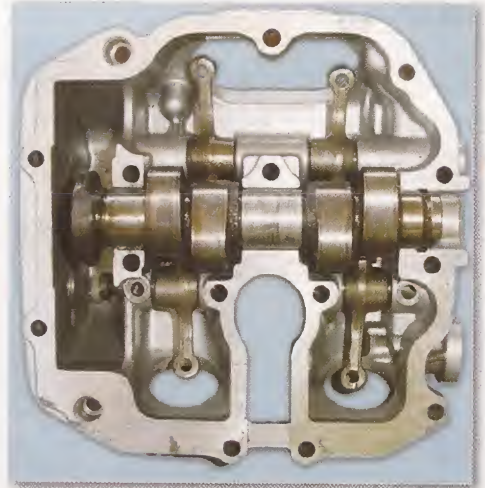
Conjunto balancín y árbol de levas en culata
